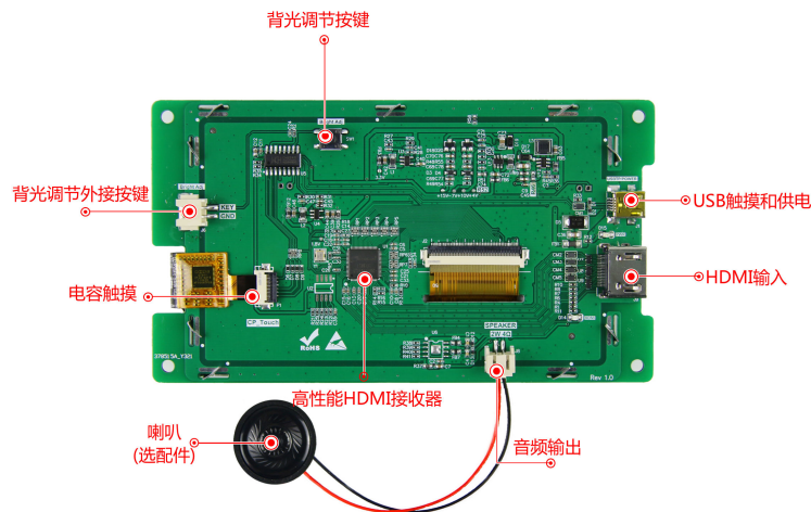
图 1-2 硬件配置图
